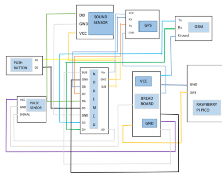
Figure 3 :Circuit Diagram
